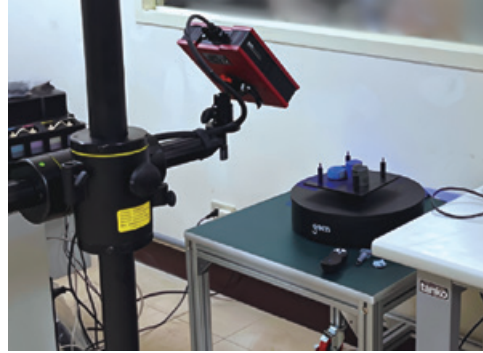
ATOS 光學掃描儀 ATOS Compact Scan
