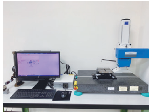
數位型輪廓儀 Digital Profiler
